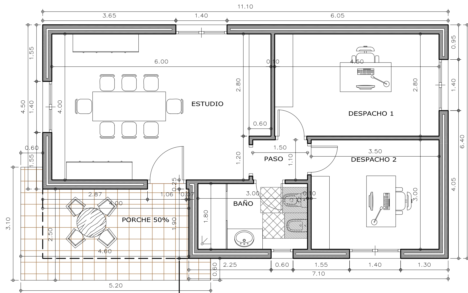
ANEXO VIVIENDA SUPERFICIE CONSTRUIDA = 71,00m 2
